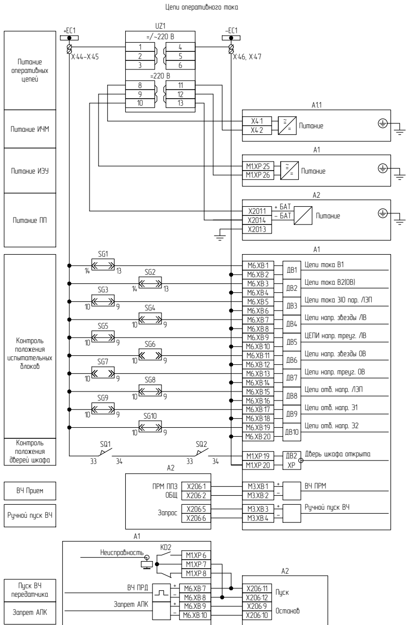
Рисунок Г.2 – Схема электрическая принципиальная (часть 2)
